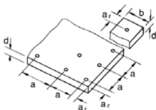
Abb. 2: R Reaktionsanker
