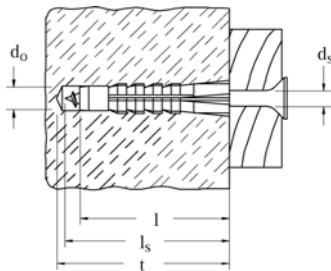
Abb. 1: UUE-Dübel
