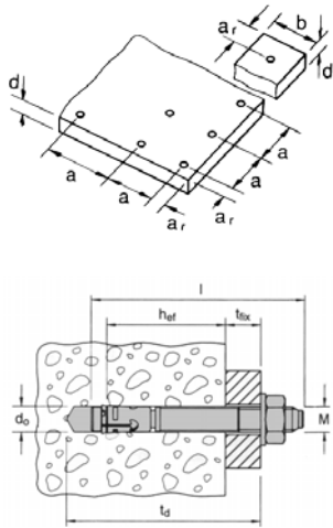
Abb. 1: Ankerbolzen FAZ
