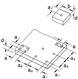
Abb. 2: FZEA-Einschlaganker
