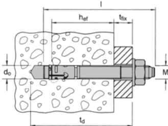
Abb. 2: Ankerbolzen FAZ II
