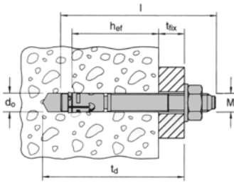
Abb. 1: Ankerbolzen FAZ
