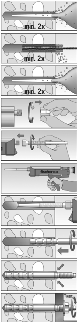
Abb. 2: Montageablauf
