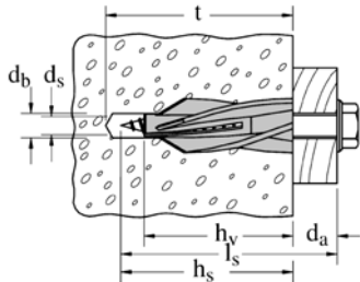
Abb. 2: GB Gasbetondübel
