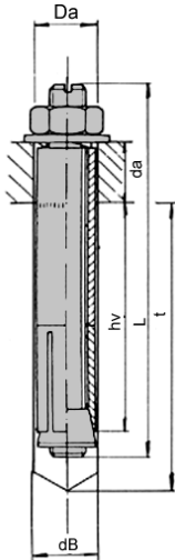
Abb. 1: AB Schwerlastanker
