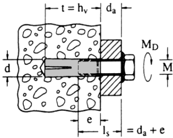
Abb. 1: EA-Einschlaganker
