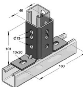
Kulma C 45 180° koodi: 08123100
