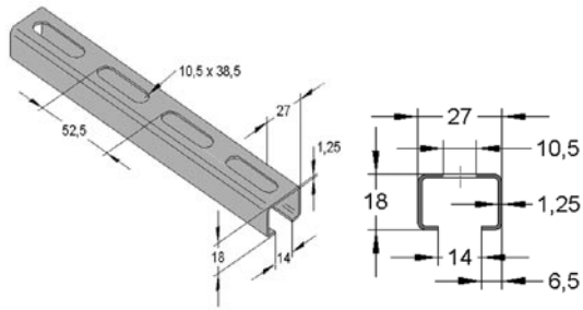
Mefa HST-kisko 27/18/1,25
