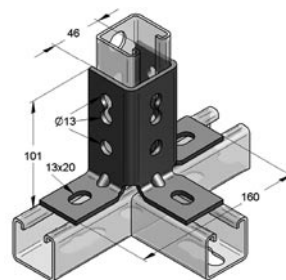
Kulma C 45 koodi: 8123000
