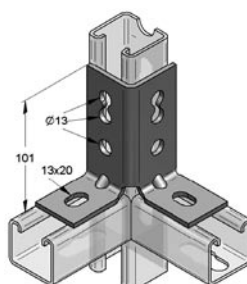
Kulma C 45 90° koodi: 08123200
